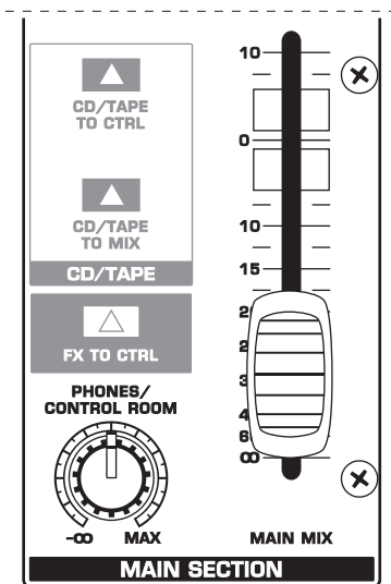
Fig. 2.10: Regulador de monitorización y fader de la mezcla principal
