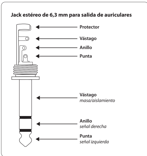
Fig. 3.4: Jack macho estéreo para auriculares
