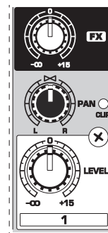
Fig. 2.3: Envíos FX / panorama / regulador de nivel
