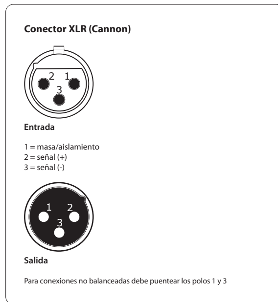
Fig. 3.1: Conexiones XLR
