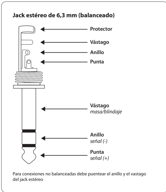
Fig. 3.3: Jack macho estéreo de 6,3 mm
