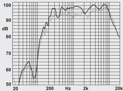
▶ CU-920HV
