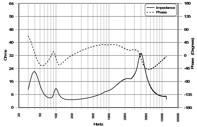
Impedance/Phase
